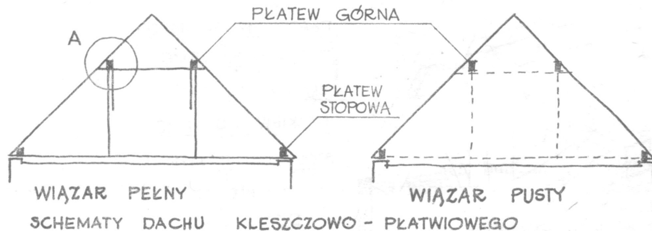
Rys. 8-13 Dach kleszczowo-płatwiowy
