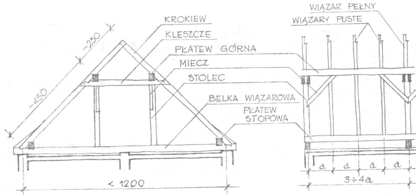
Rys. 8-13 Dach kleszczowo-płatwiowy
